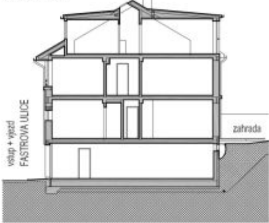
ŘEZ OBJEKTEM
