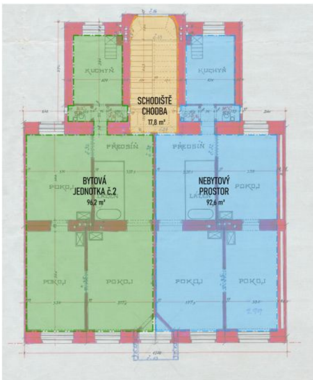
PŮDORYS 2.NP
