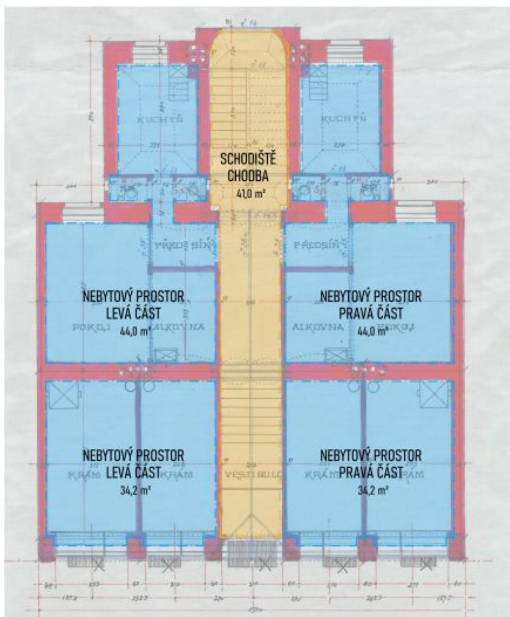
PŮDORYS 1.NP
