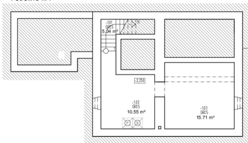
PÔDORYS 1.PP
