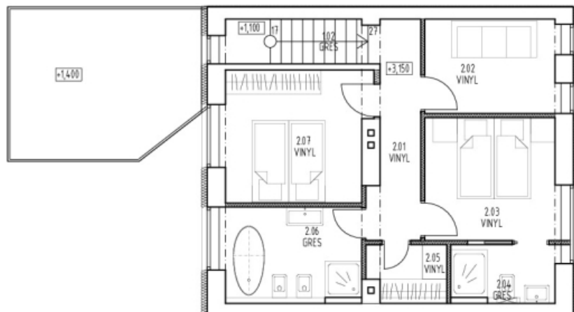
PÔDORYS 2.NP
