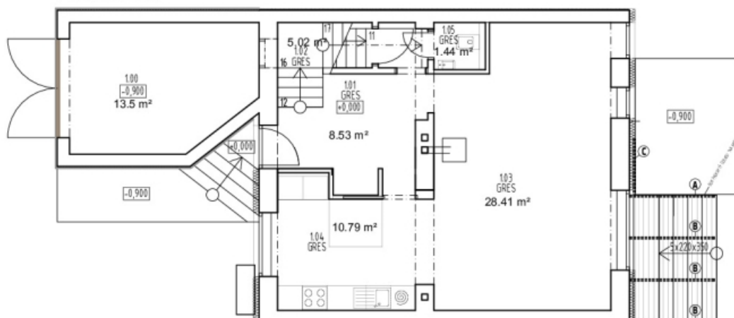
PÔDORYS 1.NP
