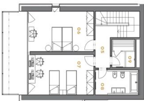
1. NP
