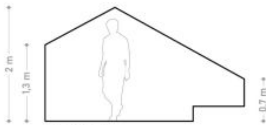
řez podkrovím
