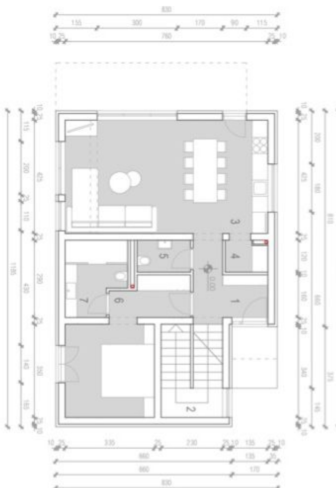
TLOCRT PRÍZEMLJA
