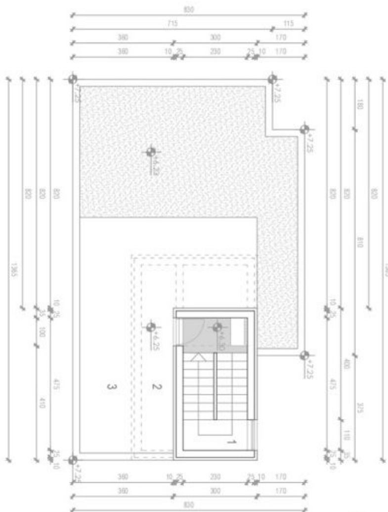
TLOCRT KROVNE TERASE
