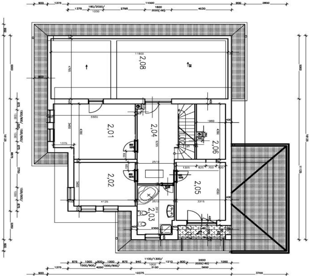
LEGENDA MIESTNOSTÍ
